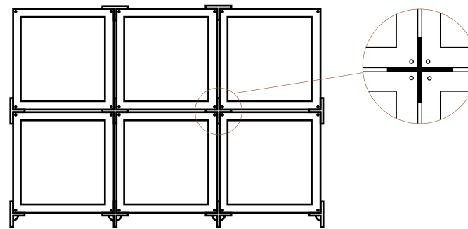
Bunke (6x Lagerung + 8x Querverbindung + 12x Verbindung Seite)
