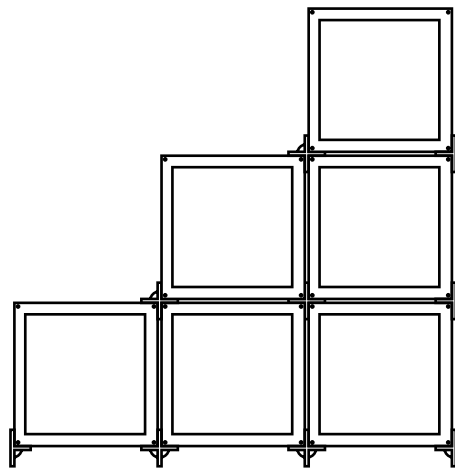
Bunke (6x Lagerung + 10x Querverbindung + 8x Verbindung Seite)
